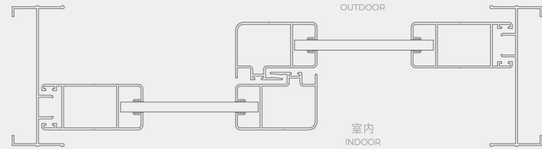
室内 INDOOR
